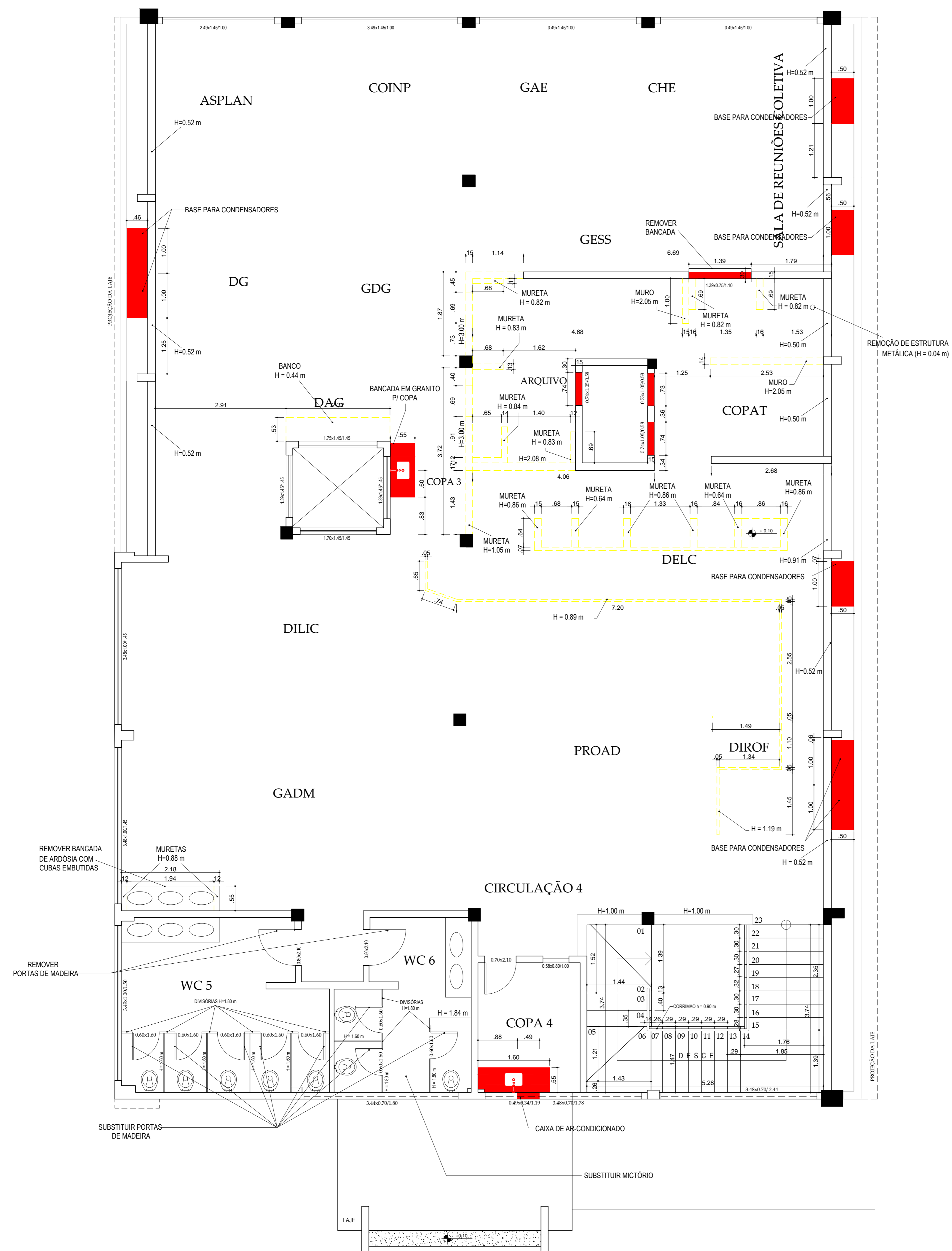
PLANTA DE REFORMA - PAV. SUPERIOR (REFEITÓRIO) ESC.: 1/50
